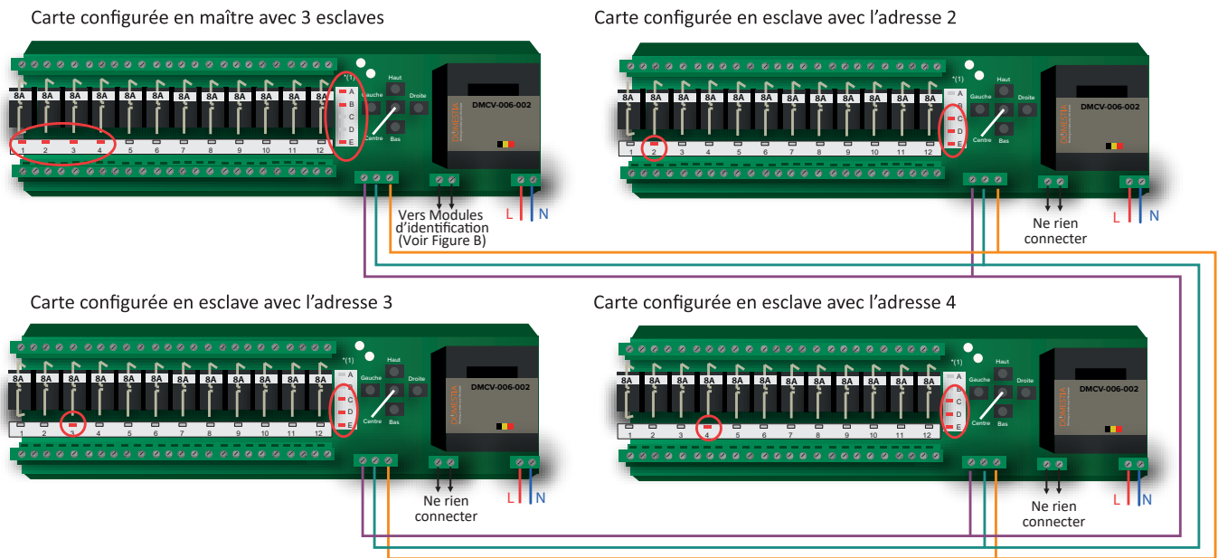
FIGURE C - Chaînage de cartes DMCV-006-002 - Exemple de raccordement de 4 cartes
