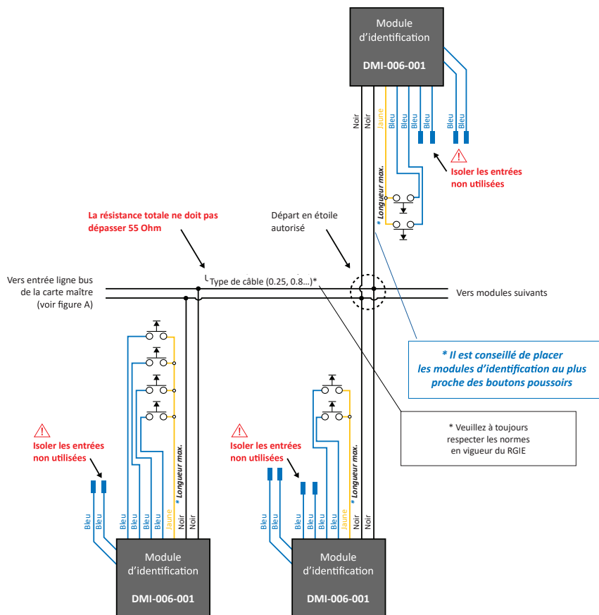
FIGURE B - Module DMI-006-001 (principe de câblage)
