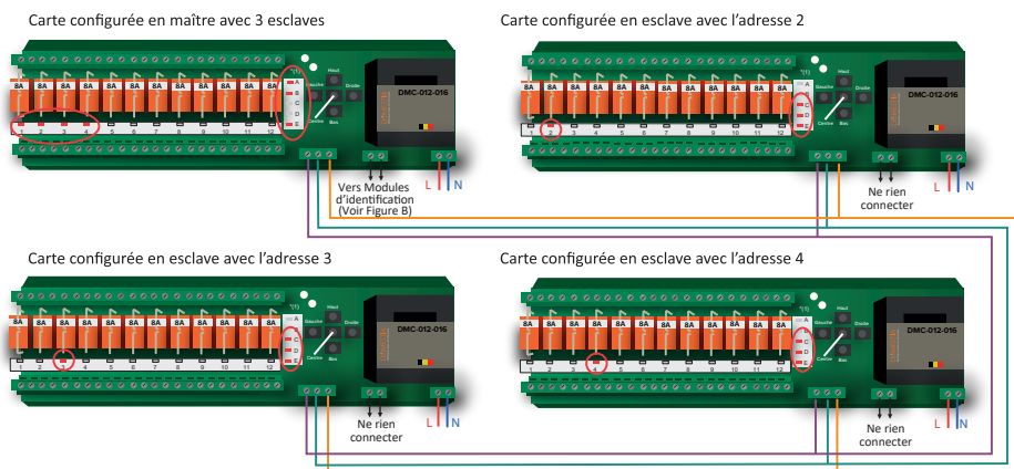
FIGURE C - Chaînage de cartes DMC-012-016 - Exemple de raccordement de 4 cartes
