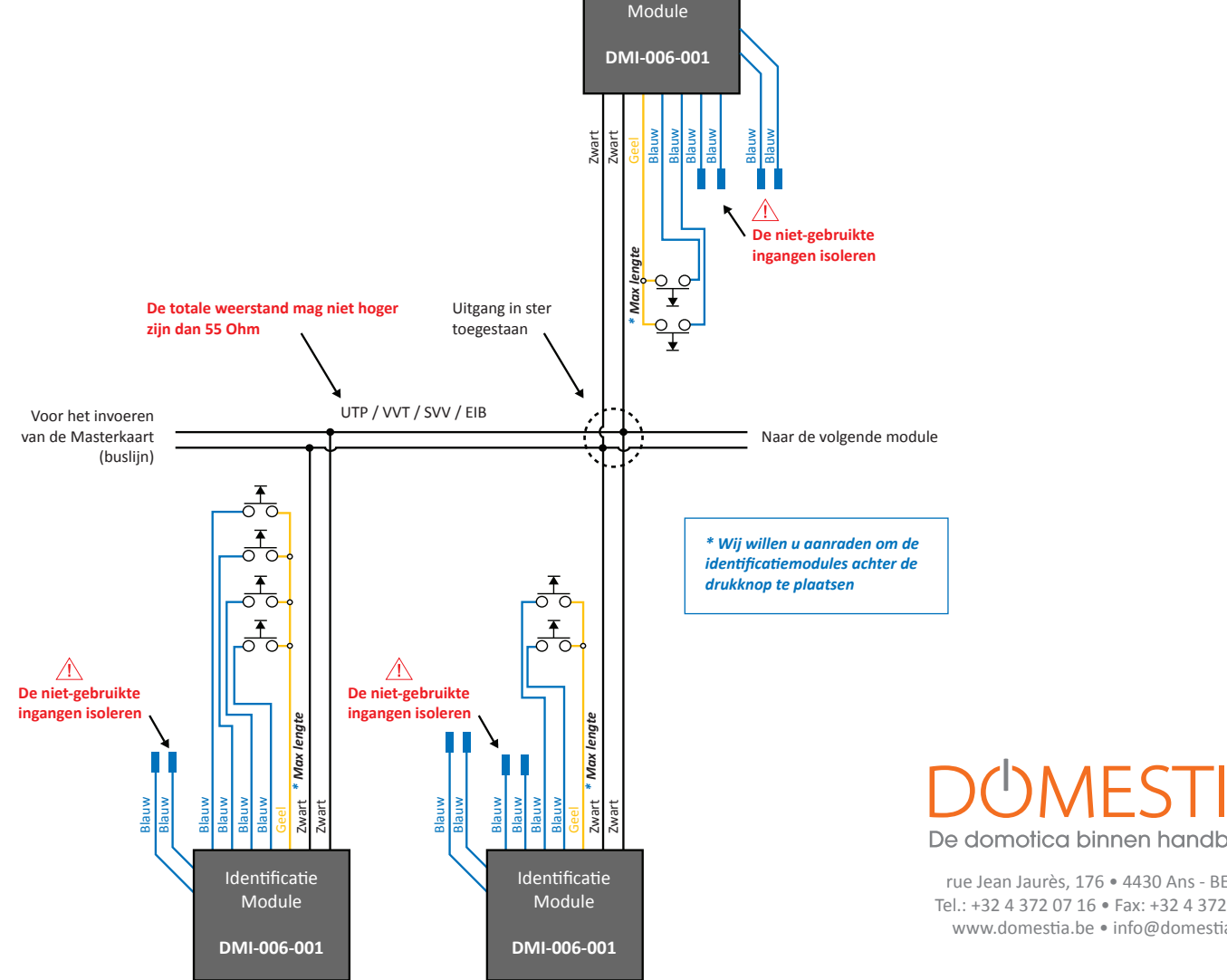
FIGUUR B - DMI-006-001 Module (bekabelingsprincipe)
